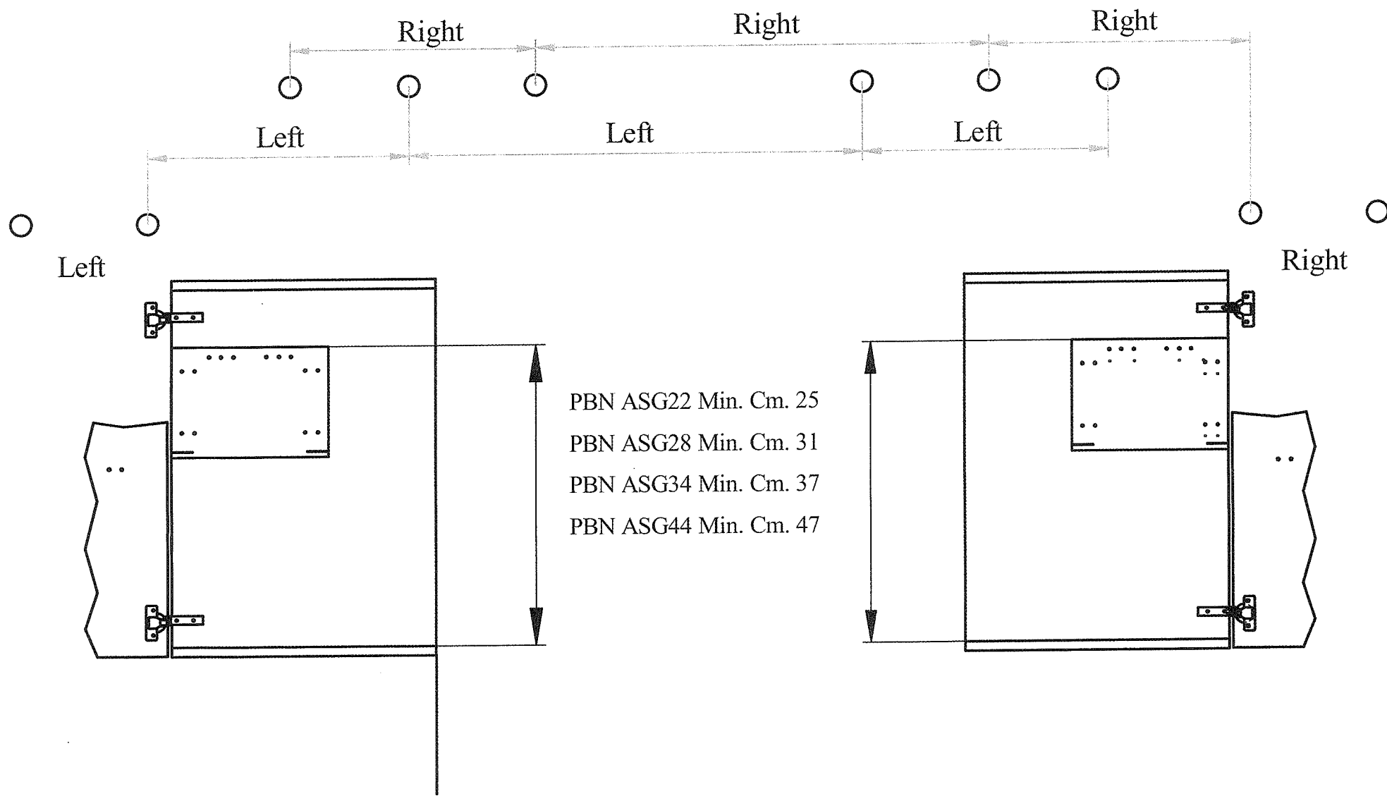
Maschera di foratura per il montaggio Drilling template for mounting
