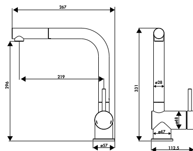
NOUVEAUTÉ RC262F09K01 Mitigeur de cuisine à bec pivotant Débit : 8,1 L/min à 3 bars Flexibles fixes
